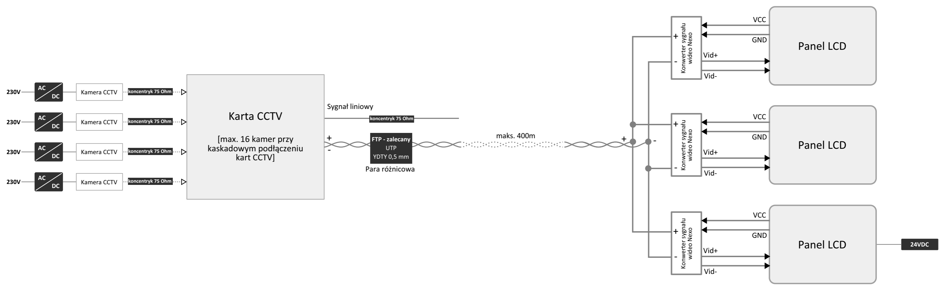
Karta CCTV - para różnicowa przy podłączeniu kilku wyświetlaczy
