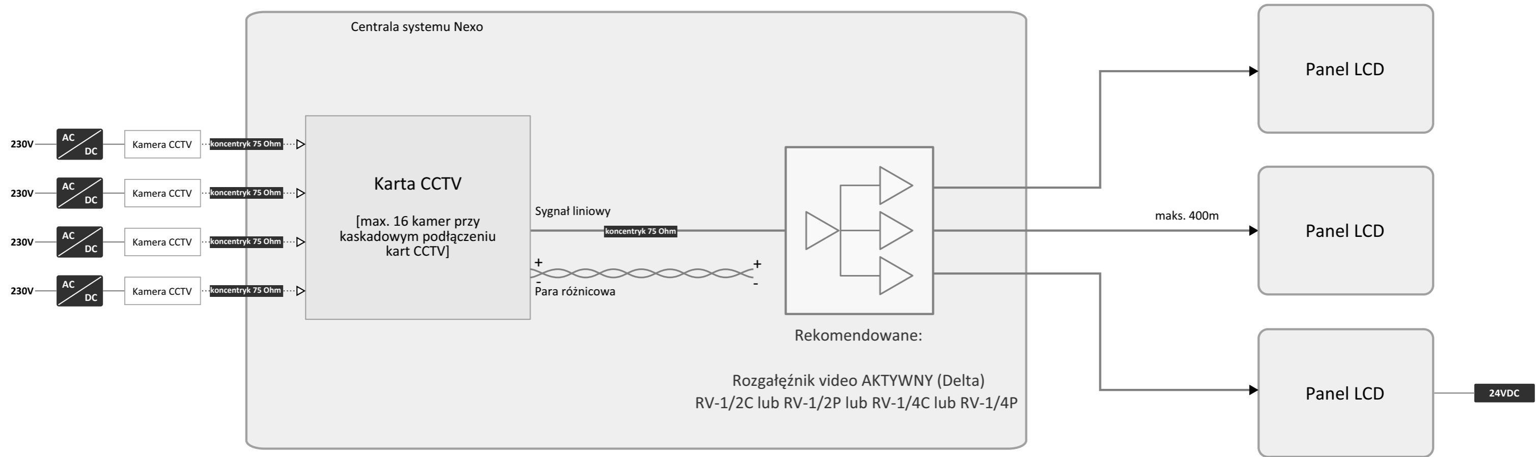
Karta CCTV - sygnał liniowy przy podłączeniu kilku wyświetlaczy
