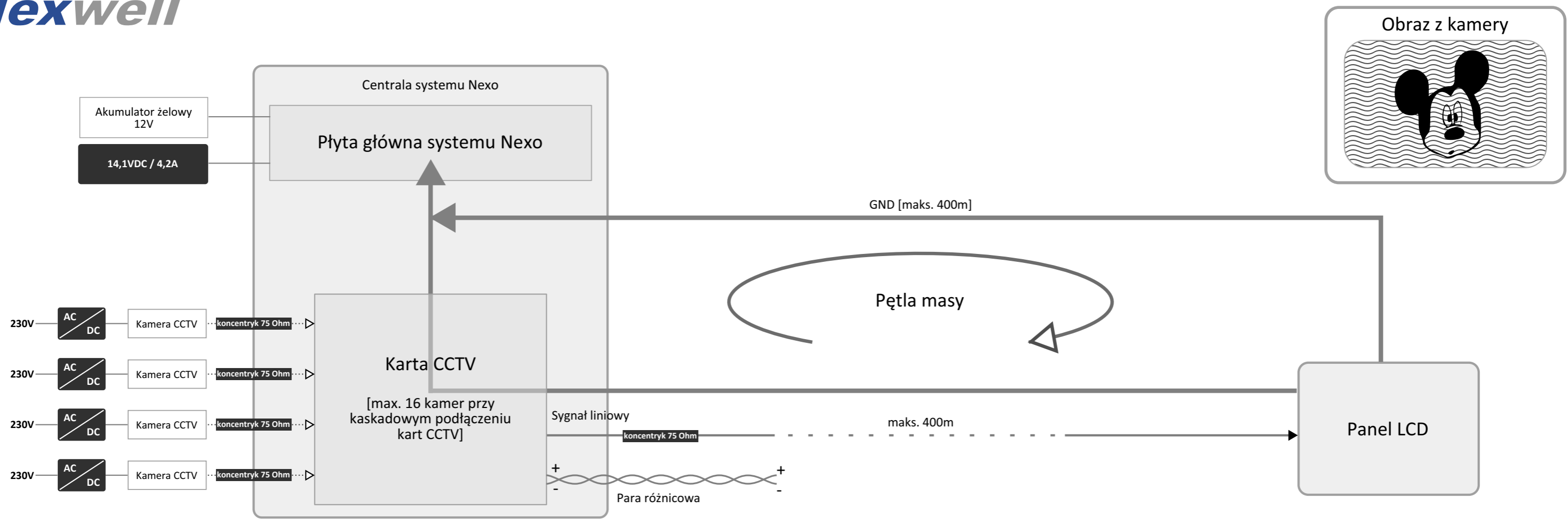
Karta CCTV - sygnał liniowy
