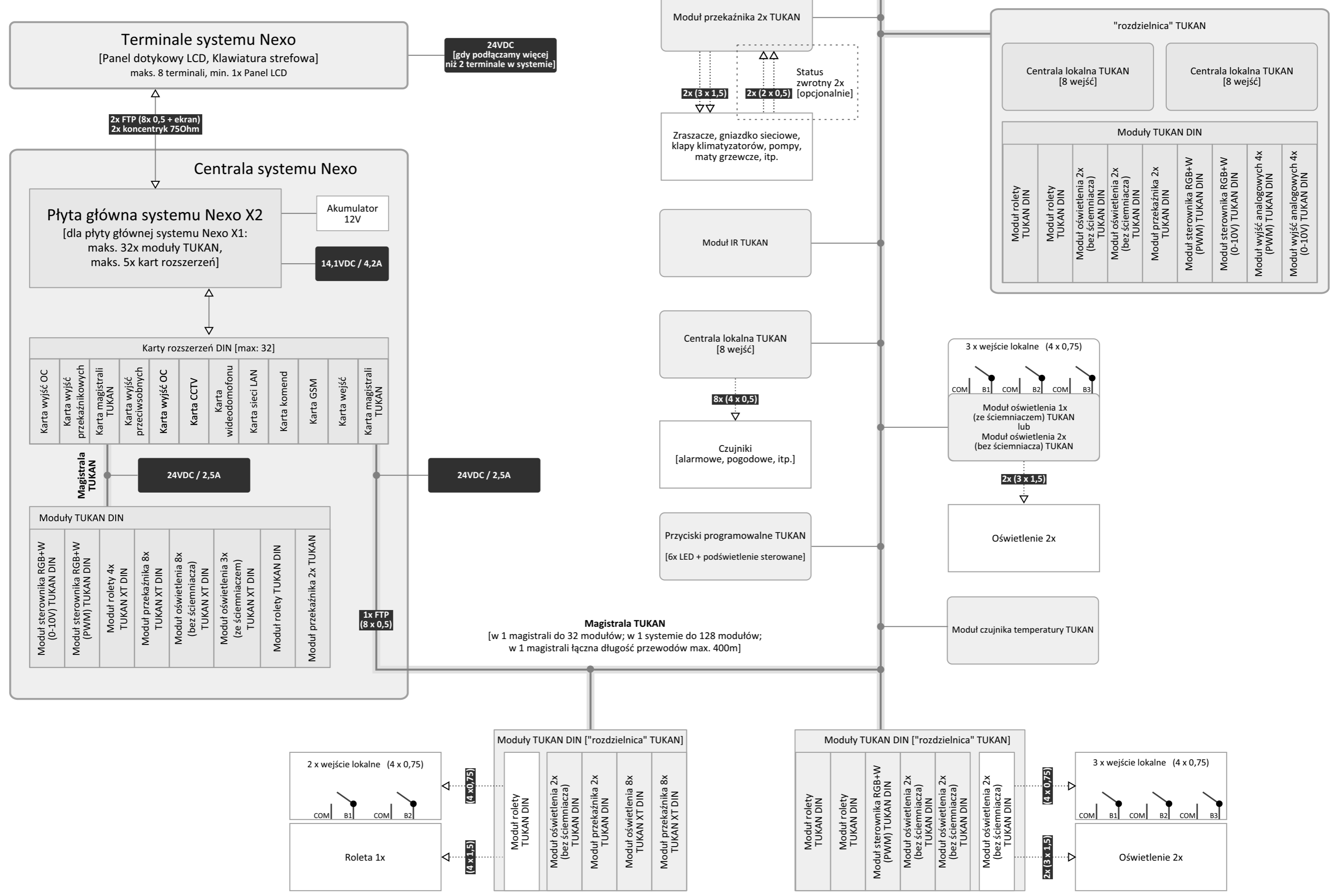
Struktura systemu Nexo - magistrala TUKAN
